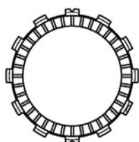
ø135.9xø124.7xø101.4x3.0mm 8PCS
