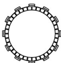
ø135.8xø124.9xø108.5x3.0mm 1PC
